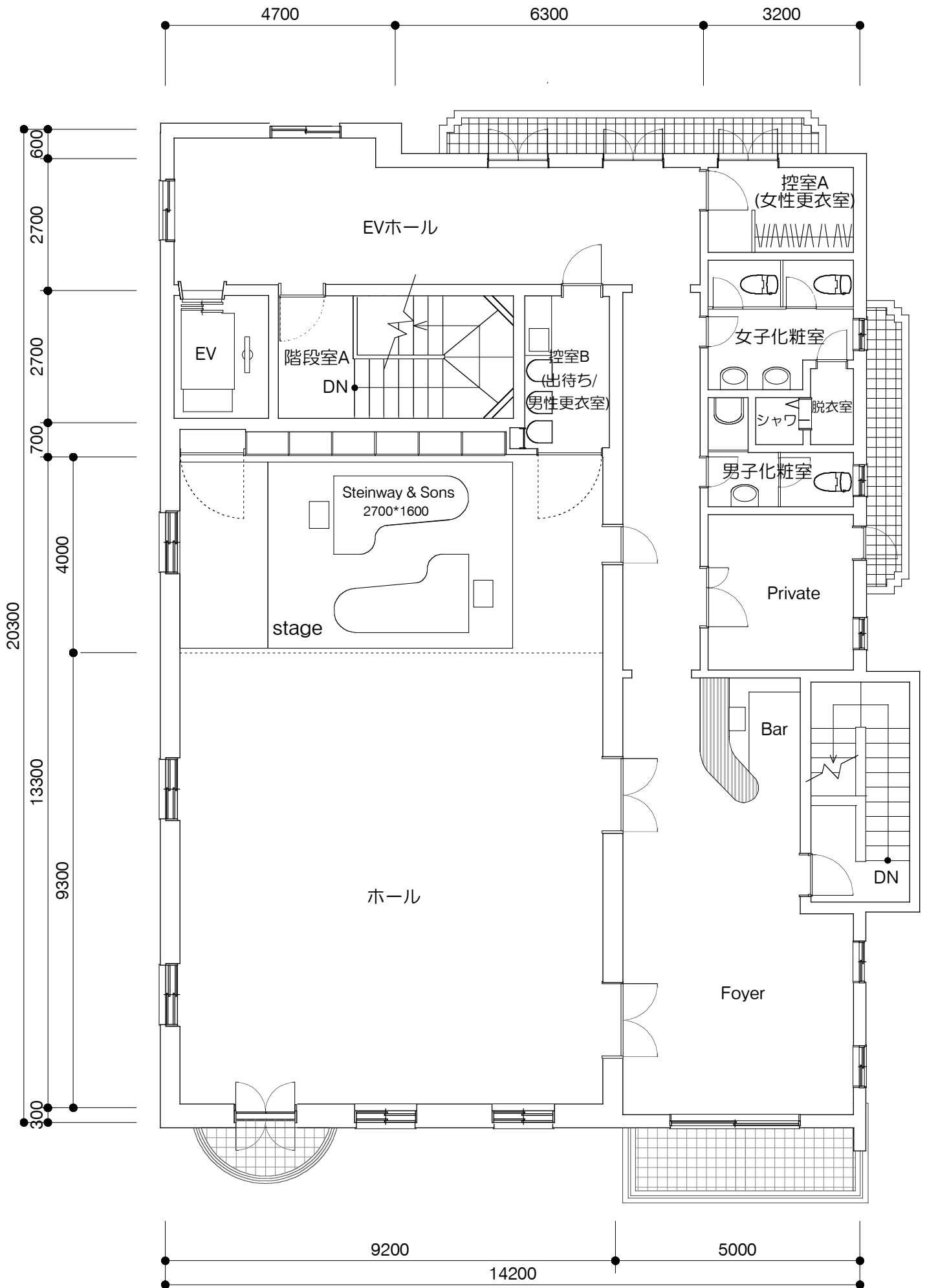
加賀町ホール●平面図 S1:100
